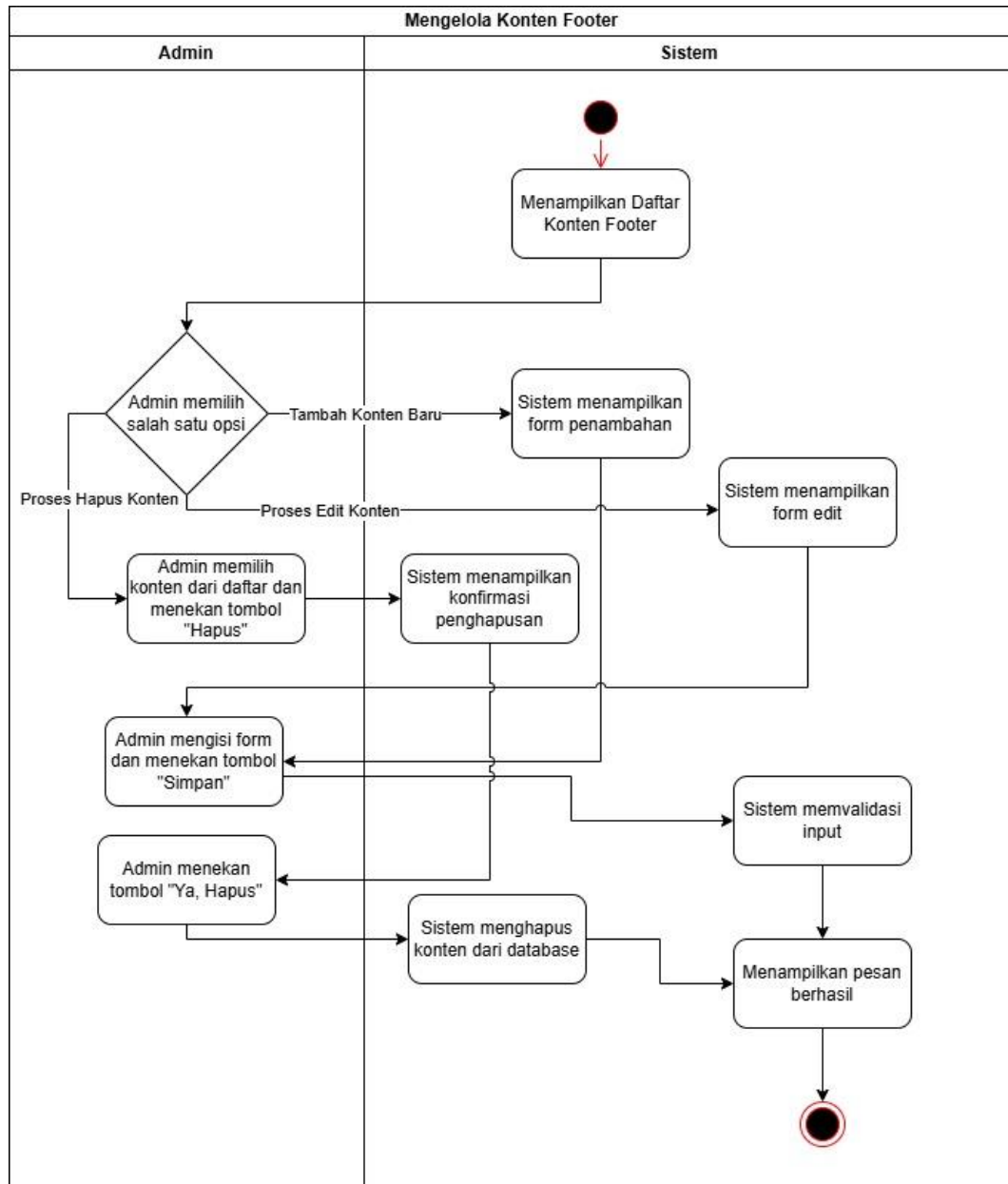
Gambar 1. 7 Activity Diagram Mengelola Konten Footer
