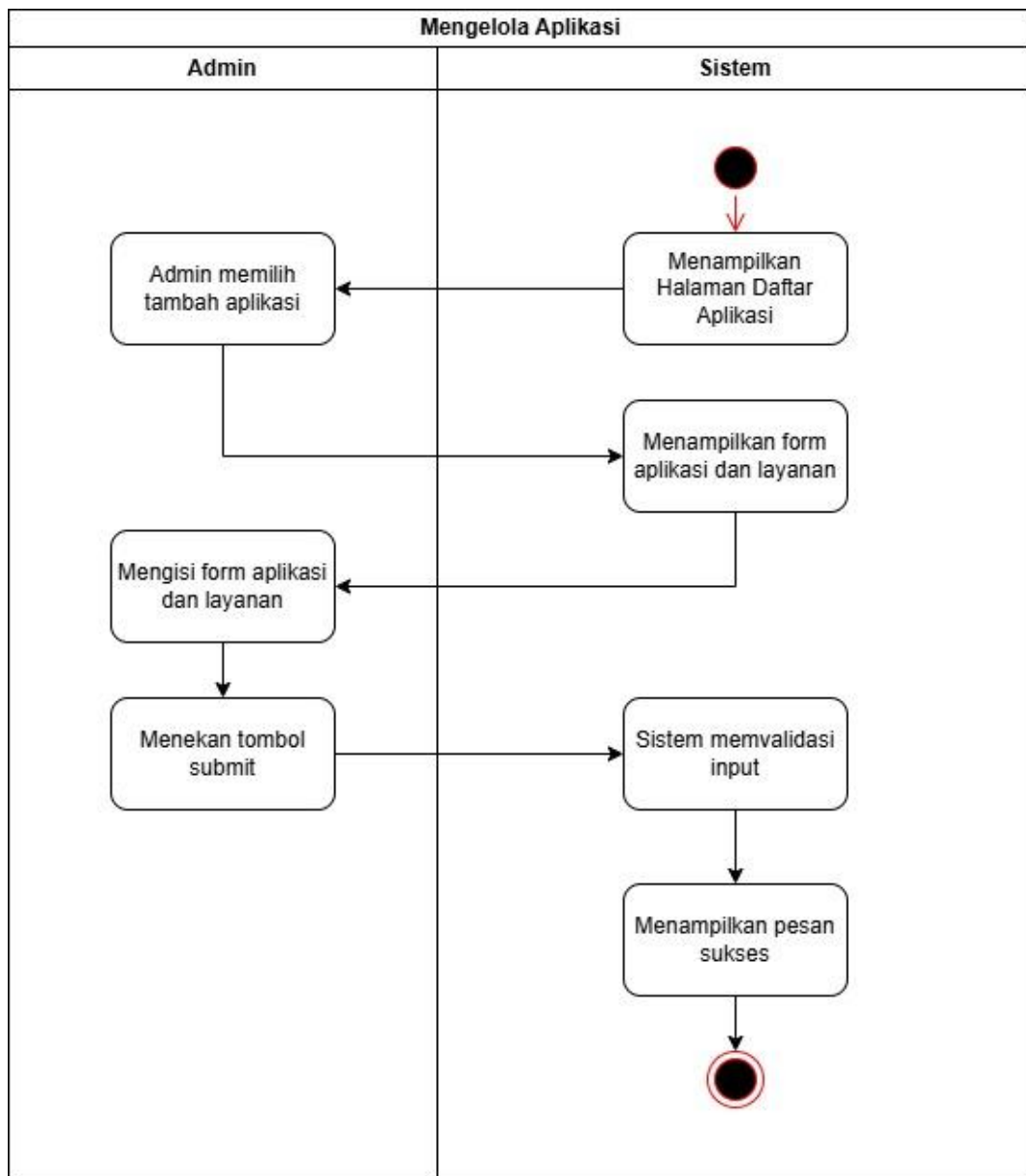
Gambar 1. 6 Activity Diagram Mengelola Aplikasi
